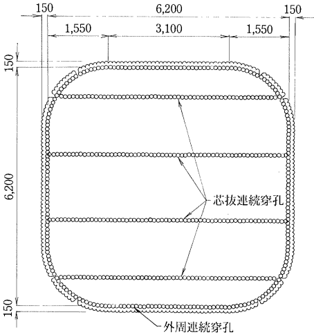
図-4 スロット配置図
